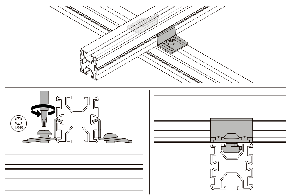
Rys. 44: Przykręcanie łącznika krzyżowego
