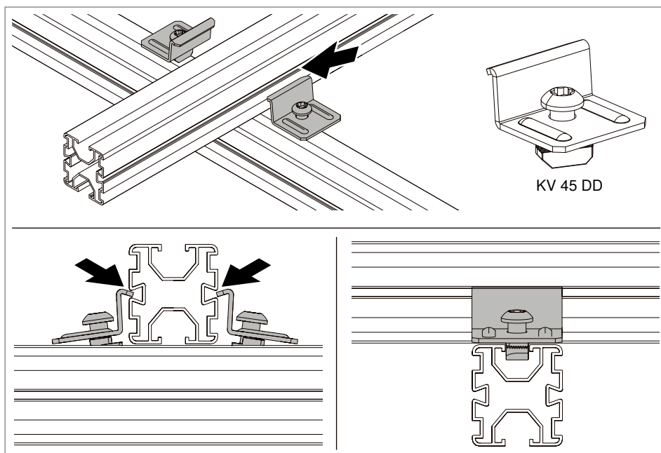
Rys. 43: Umieszczanie łącznika krzyżowego
